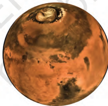
Fig. 13.6: Mars
