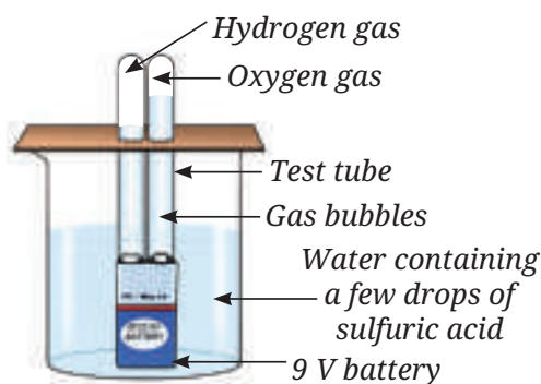
(d) Gases collected in the test tubes
